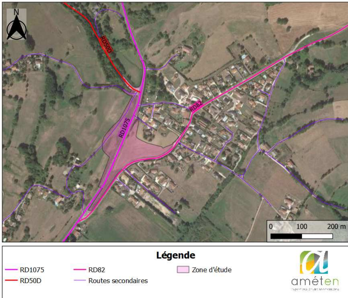
Figure 2 : Contexte au droit du projet de carrefour giratoire de l'Arsenal
